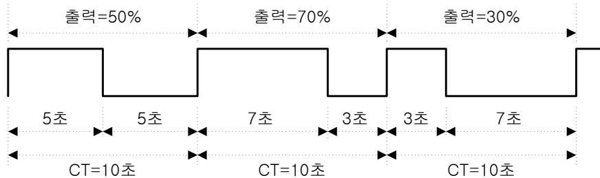
(그림 3 : CT = 10초의 경우 제어출력 동작 예)
