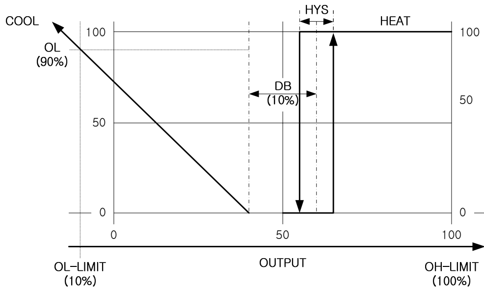
(그림 7 : HEAT = ON/OFF, COOL = PID 제어인 경우 예)
