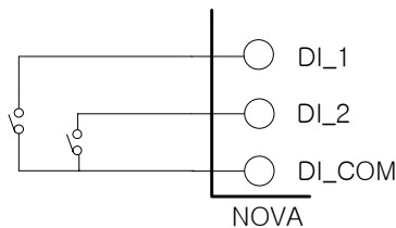
▲ RELAY 접점입력의 경우
