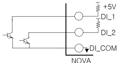
▲ TRANSISTOR 접점입력의 경우
