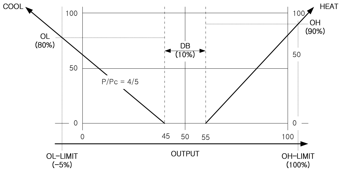
(그림 6 : HEAT과 COOL이 모두 PID 제어인 경우 예)
