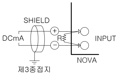
(다) 직류전류 입력(DC CURRENT INPUT)
