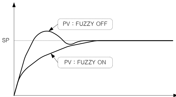
(그림 5 : FUZZY 기능에 의한 OVER SHOOT 억제)
