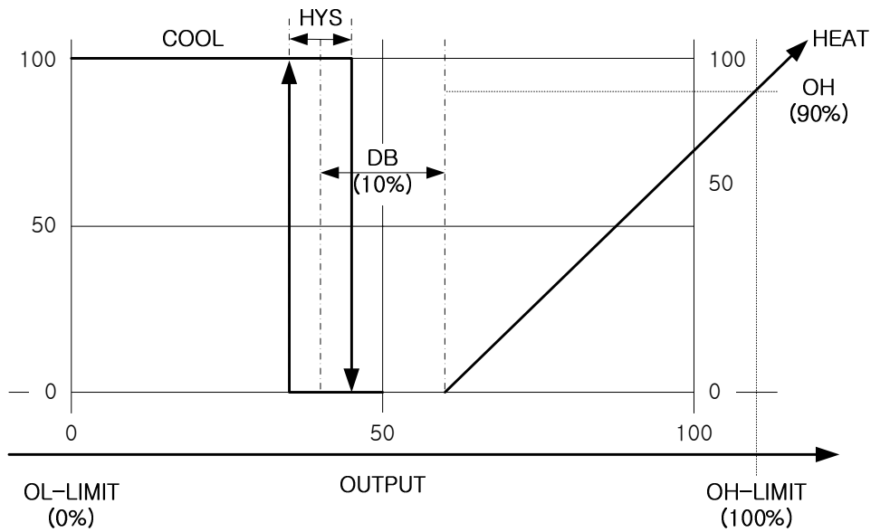
(그림 8 : HEAT = PID, COOL = ON/OFF 제어인 경우 예
