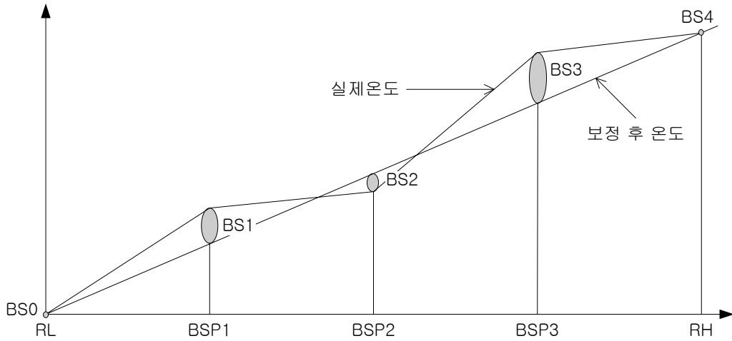
(그림 1 : 구간별 입력 보정(BIAS) 설정 예)
