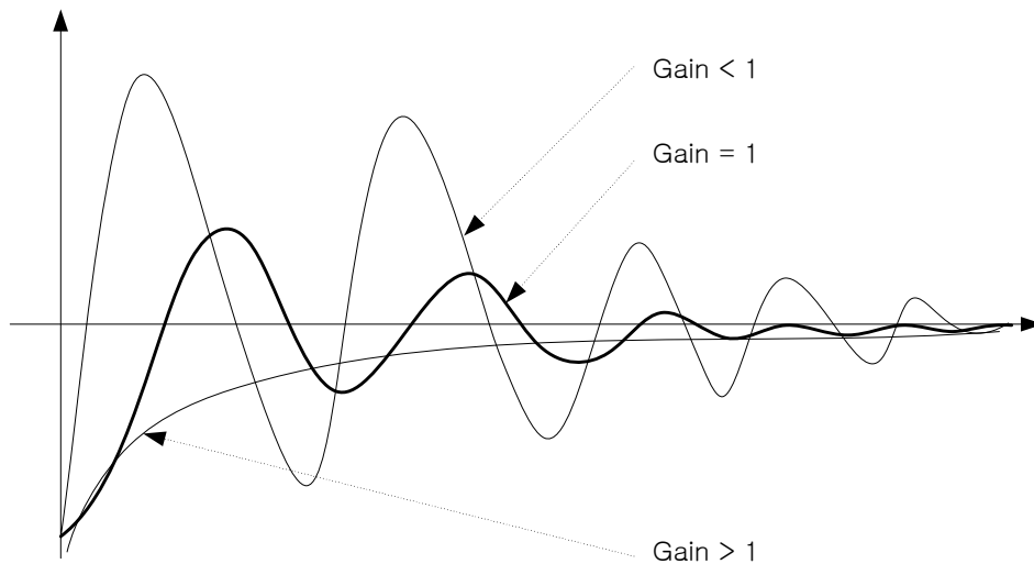
(그림 10 : AT GAIN)
