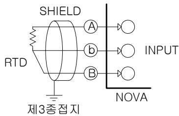
(가) 측온저항체 입력(RTD INPUT)
